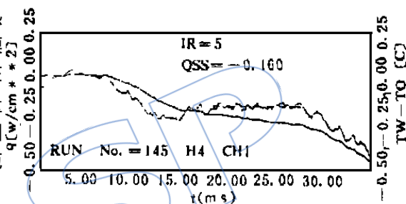
图 3 壁面热通量随时间的变化
